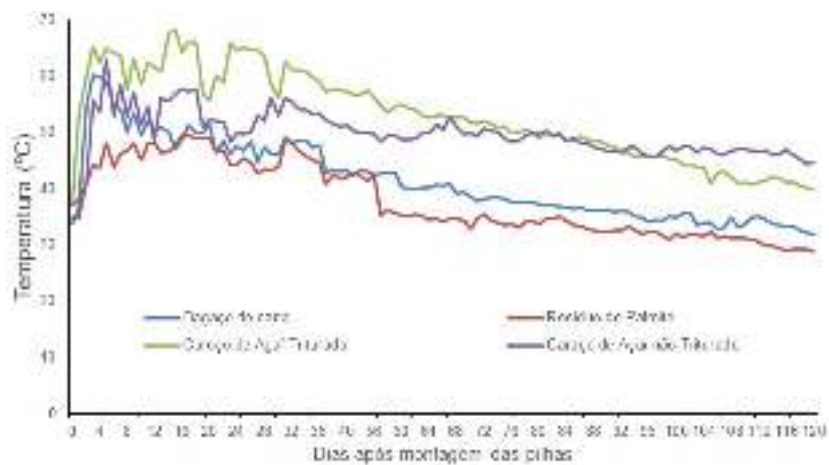
Figura 1. Temperatura observada nas diferentes pilhas de compostagem.
